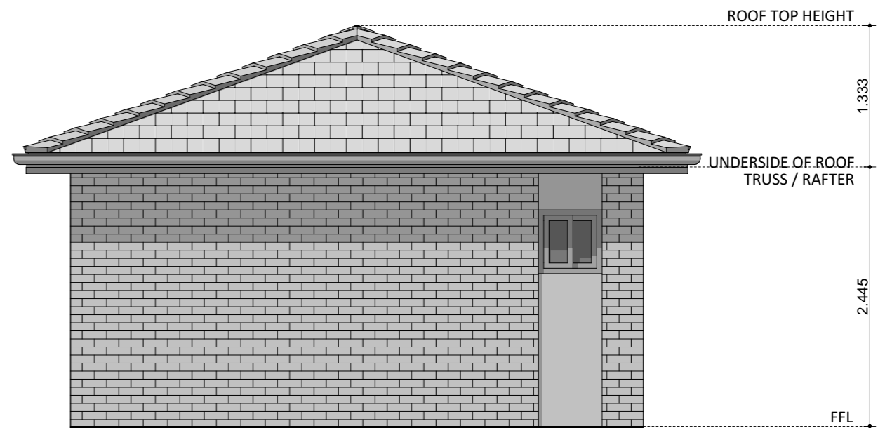
ELEVATION 04
