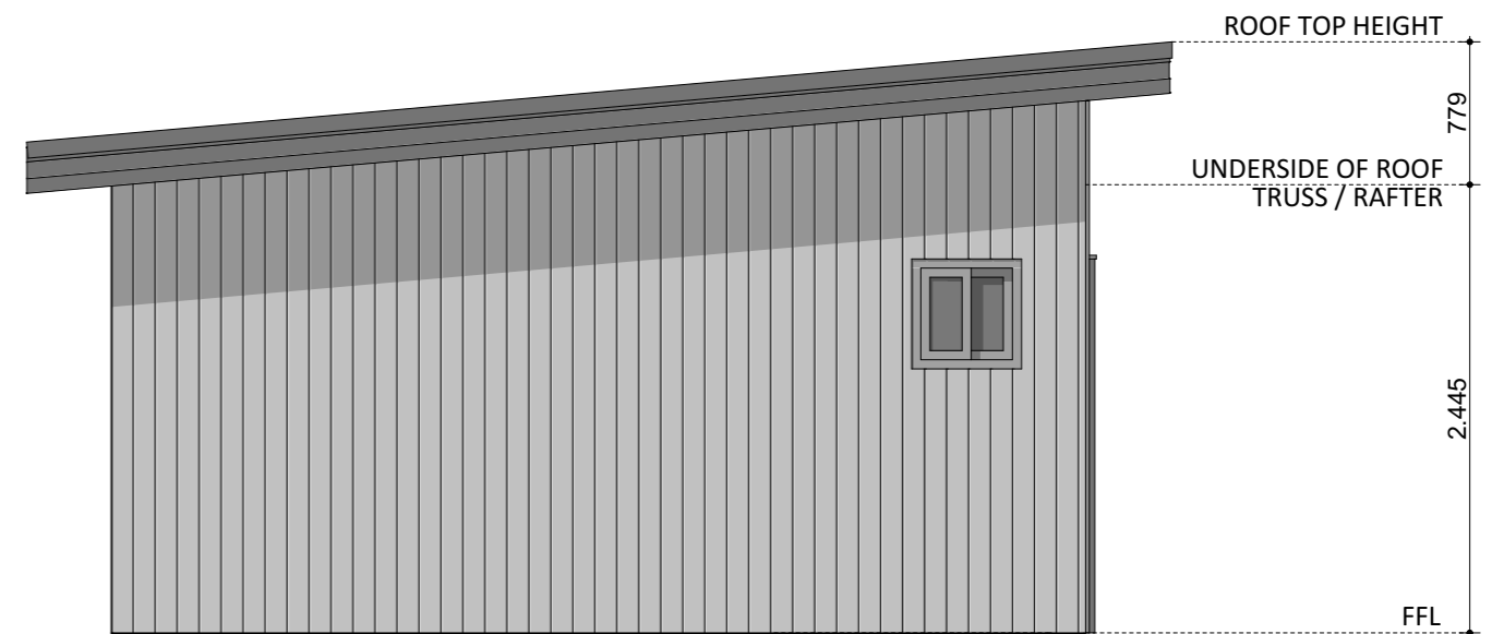
ELEVATION 04
