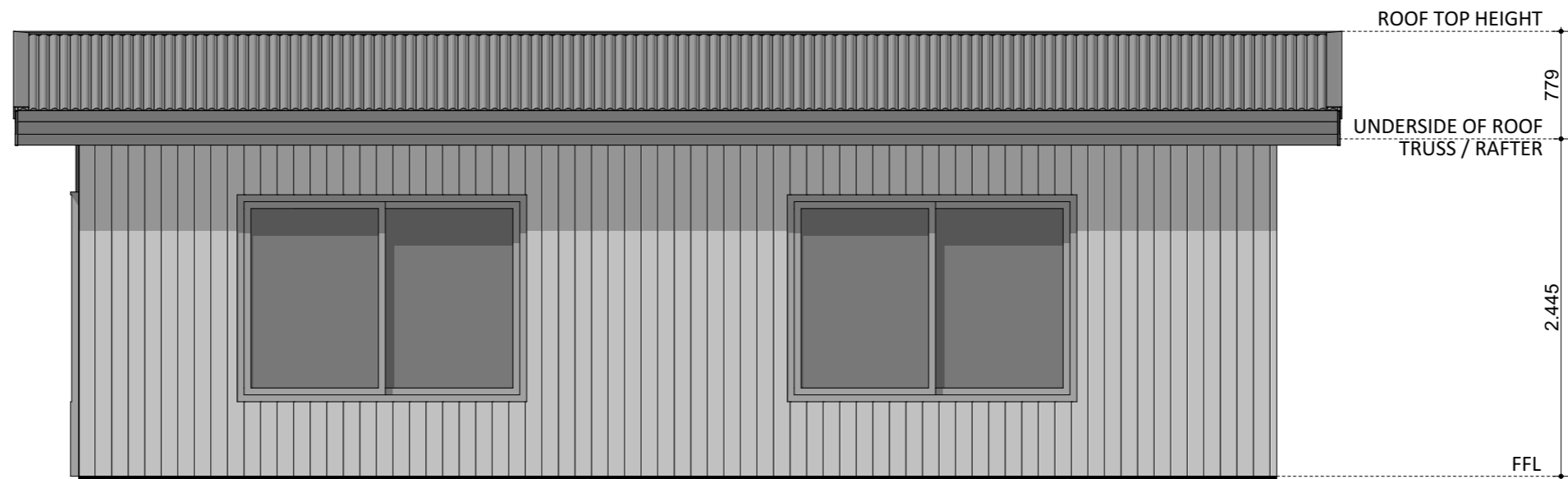
ELEVATION 01
