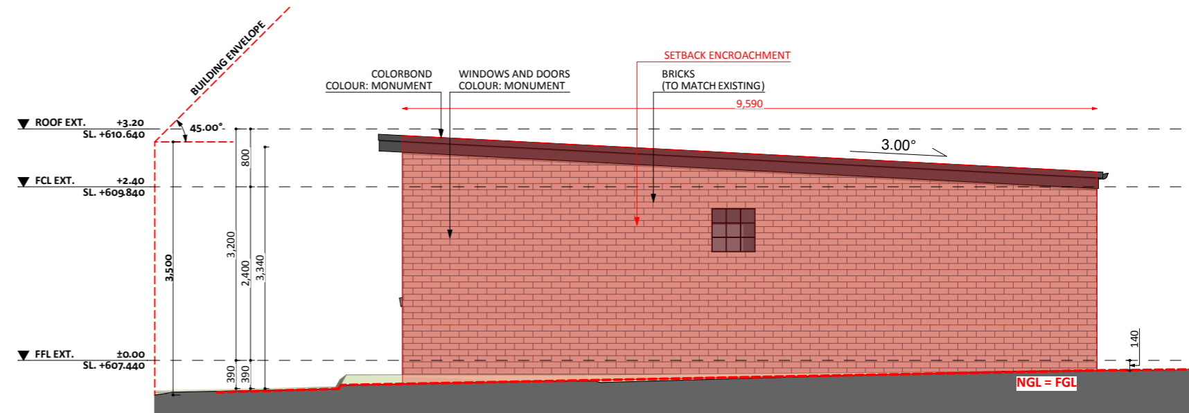
ELEVATION 04
