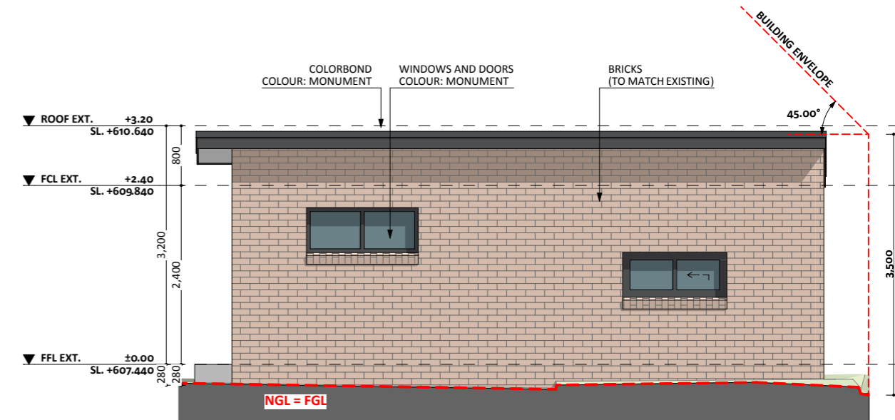
ELEVATION 02
