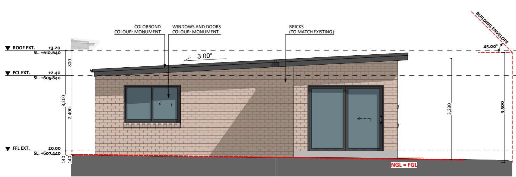
ELEVATION 01
