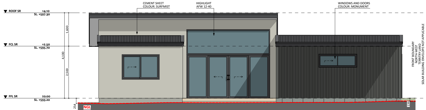
ELEVATION 01
