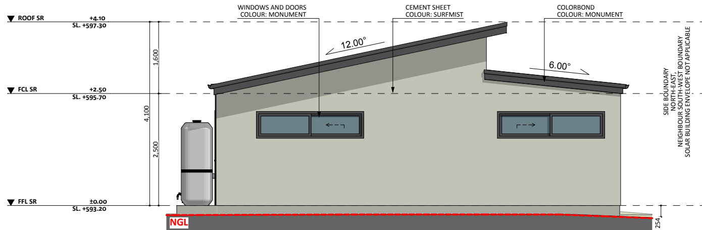
ELEVATION 02
