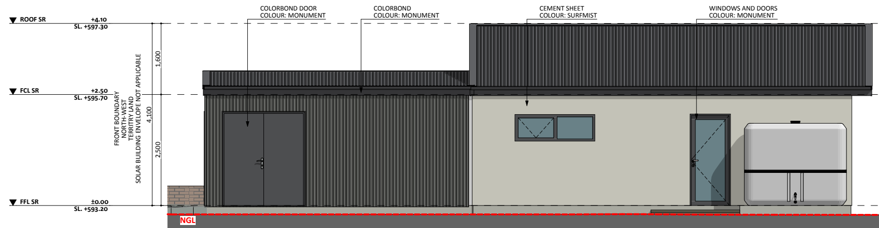
ELEVATION 04
