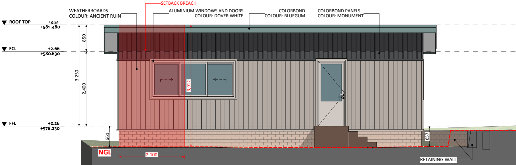
ELEVATION 01
