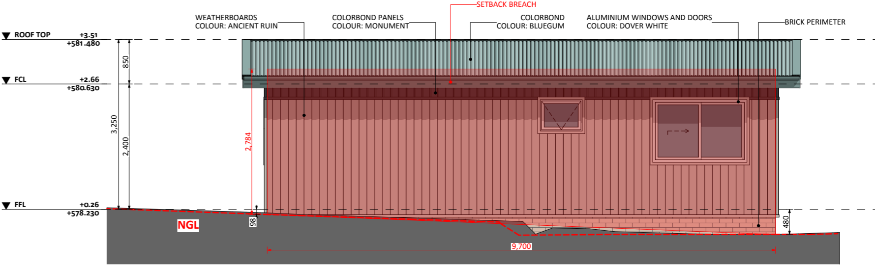
ELEVATION 04
