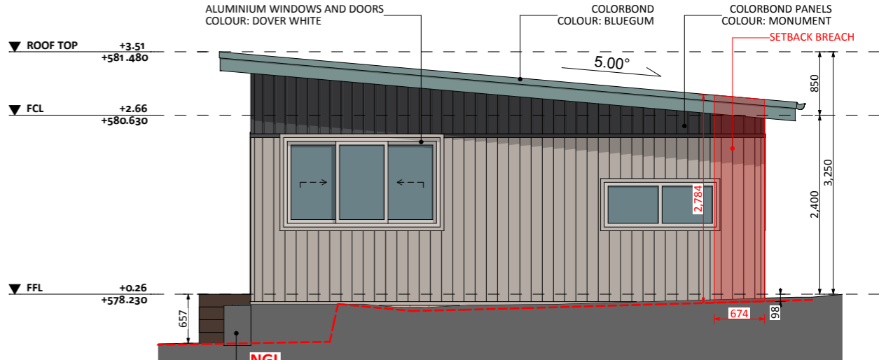
ELEVATION 02
