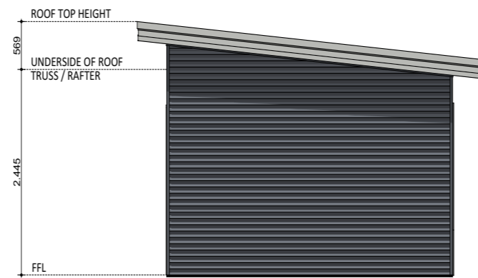
ELEVATION 02
