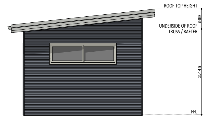
ELEVATION 04
