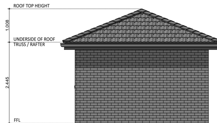
ELEVATION 02
