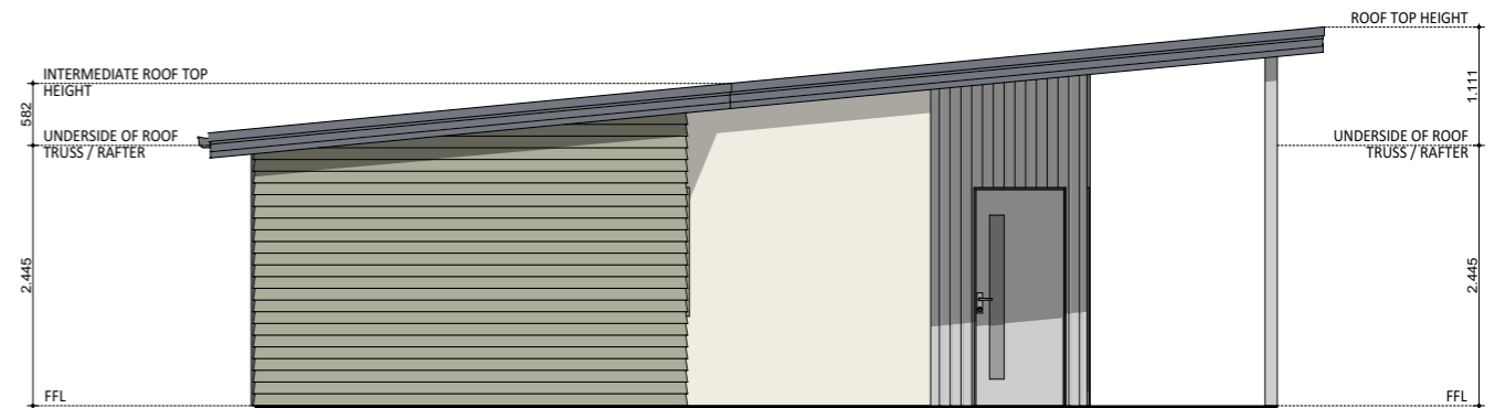
ELEVATION 02
