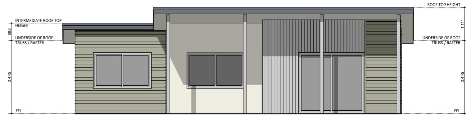
ELEVATION 01
