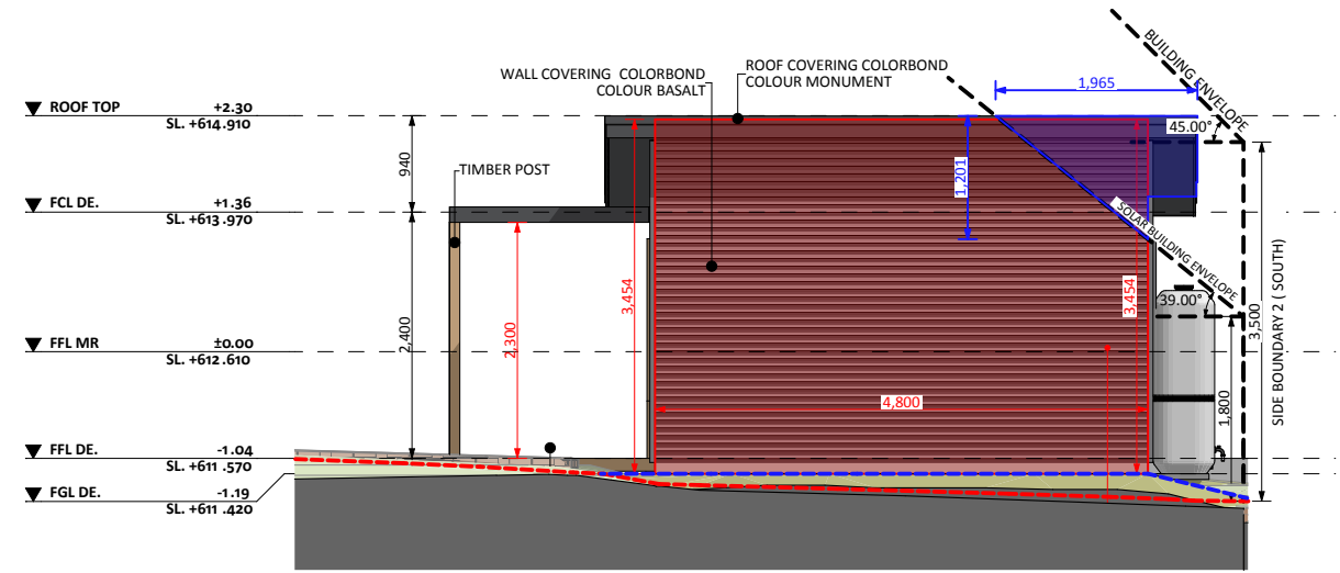
ELEVATION 02
