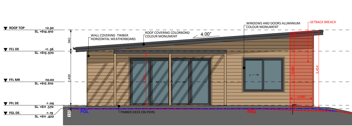
ELEVATION 01
