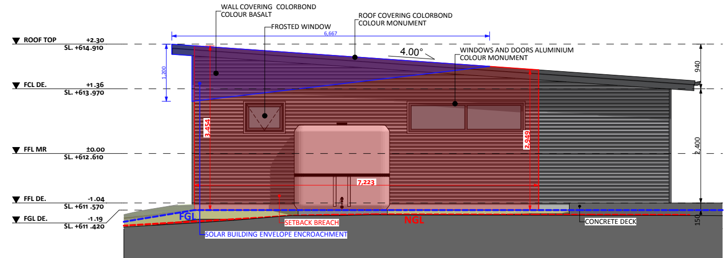
ELEVATION 04
