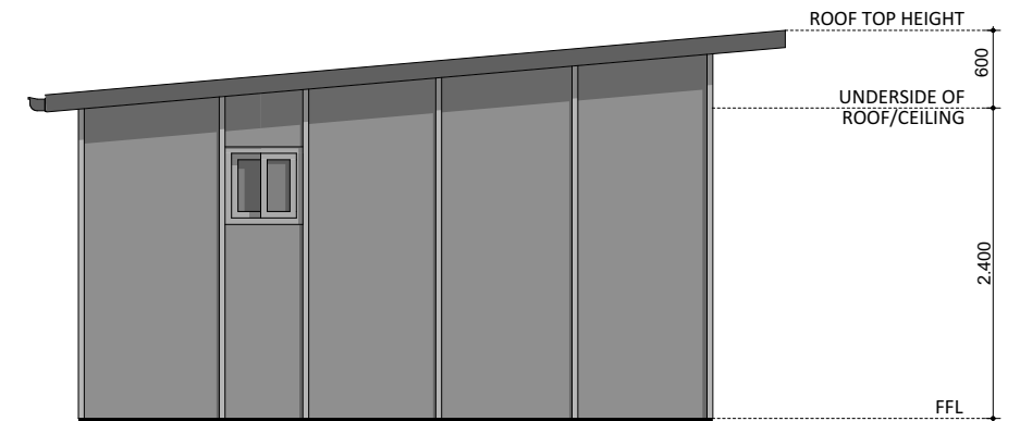
ELEVATION 04
