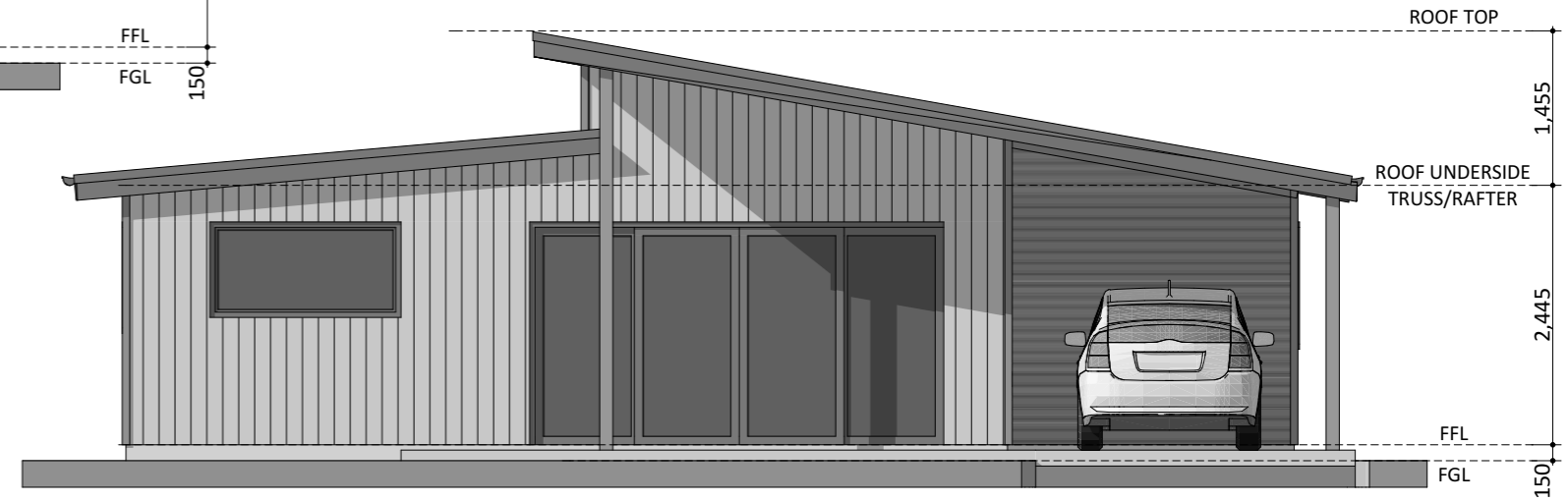
ELEVATION 2
