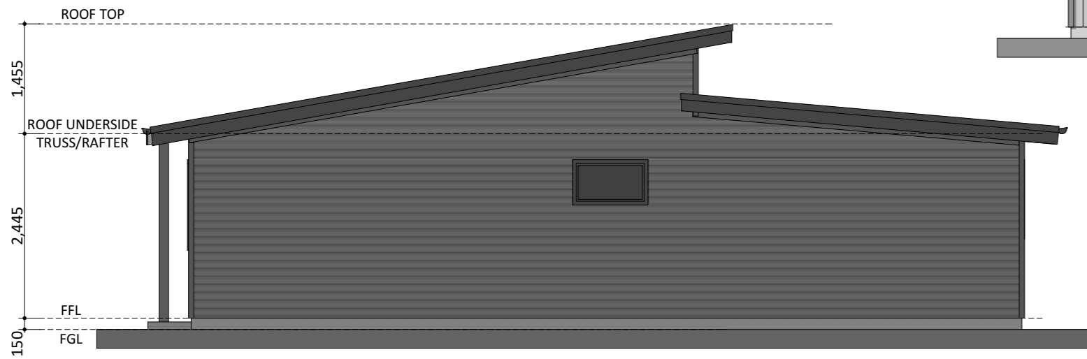
ELEVATION 3
