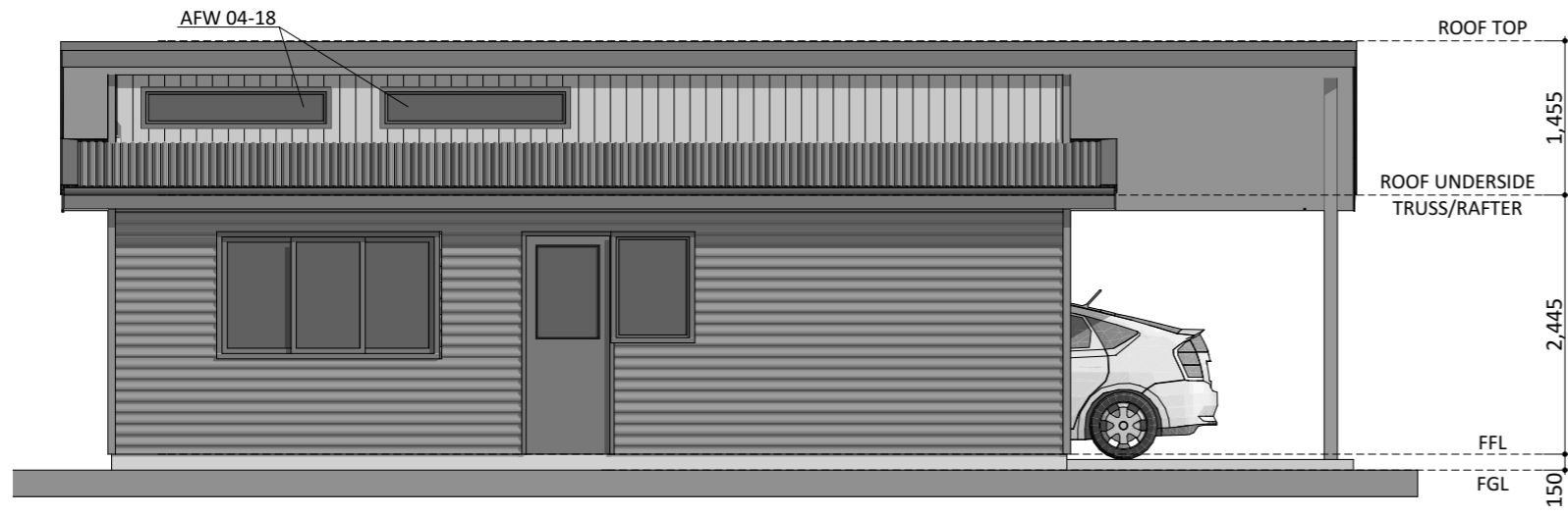
ELEVATION 1
