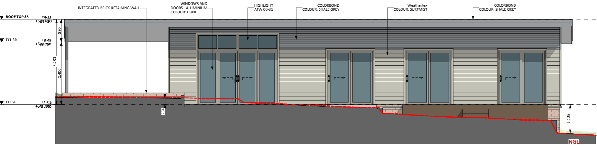
ELEVATION 01
