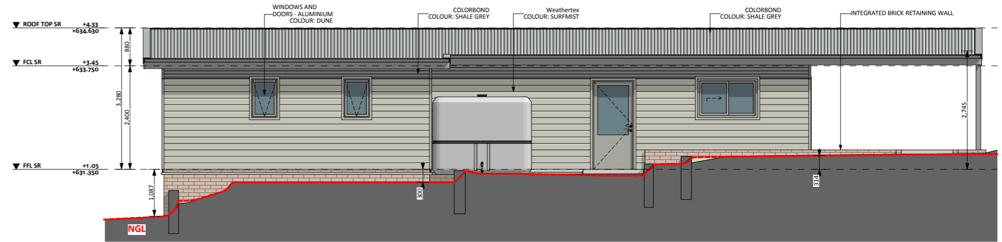
ELEVATION 04
