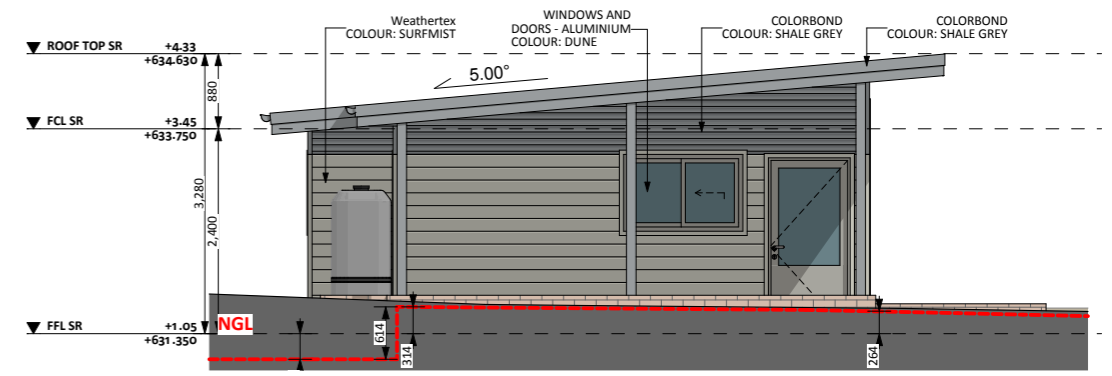
ELEVATION 02
