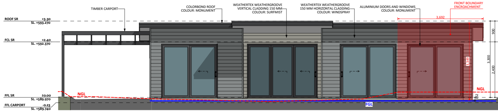
ELEVATION 01
