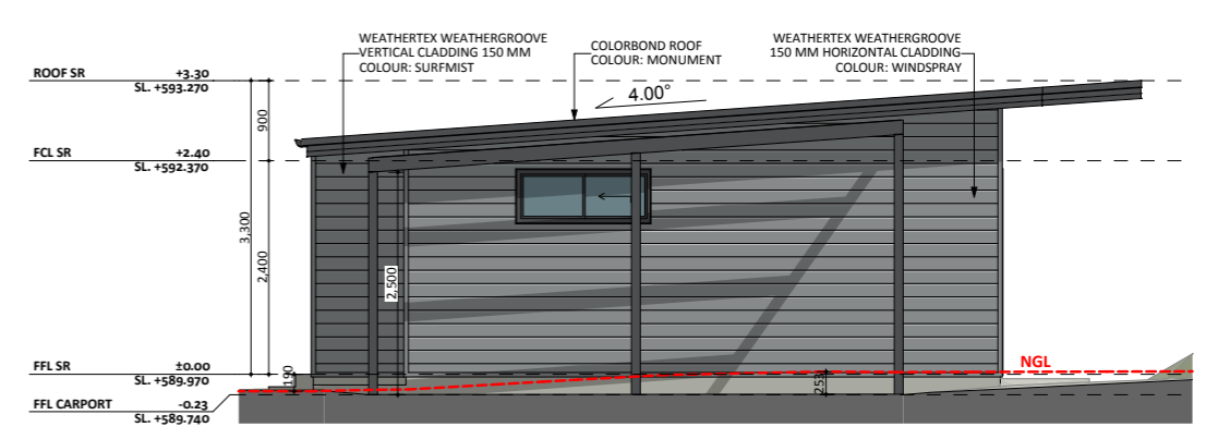
ELEVATION 02
