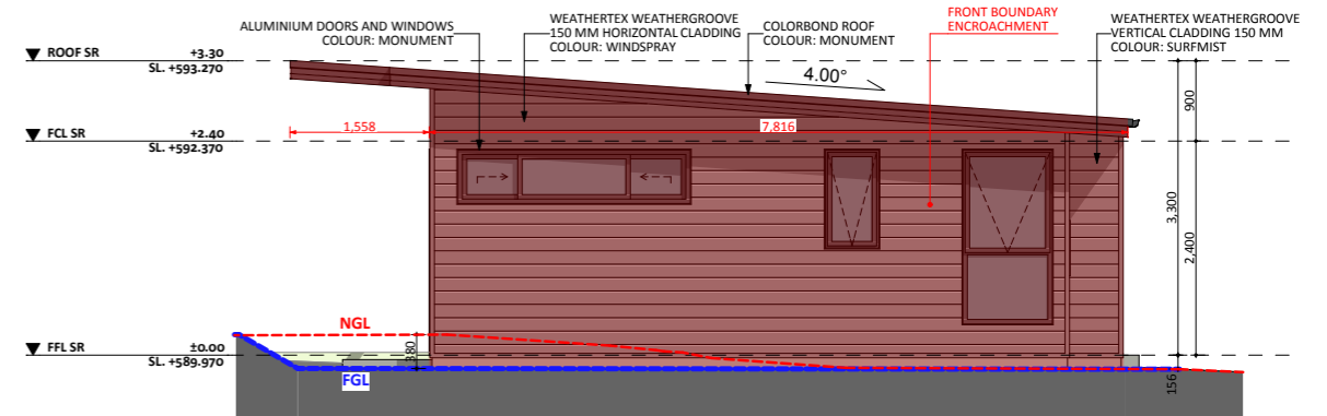
ELEVATION 04
