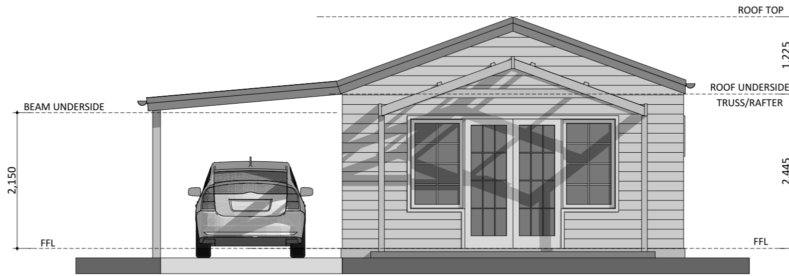
ELEVATION 01
