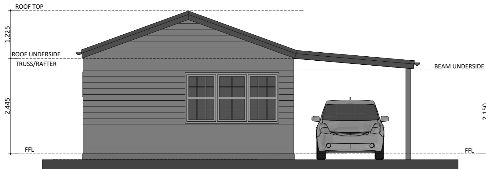
ELEVATION 02
