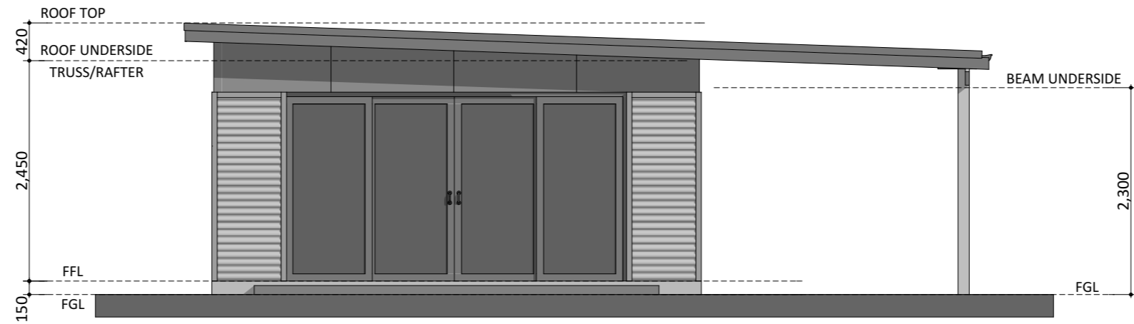
ELEVATION 01
