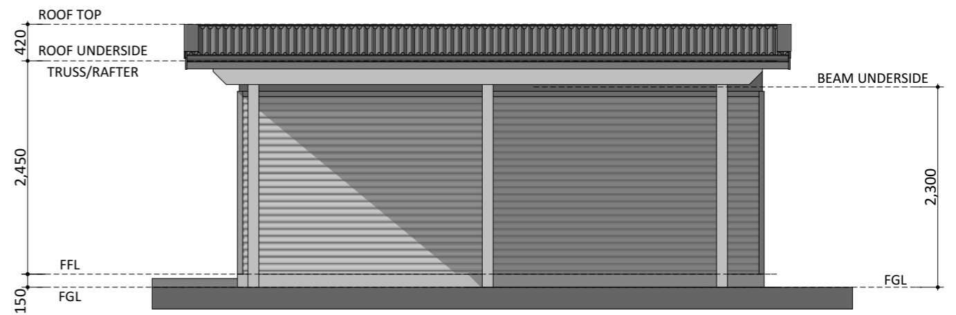
ELEVATION 04
