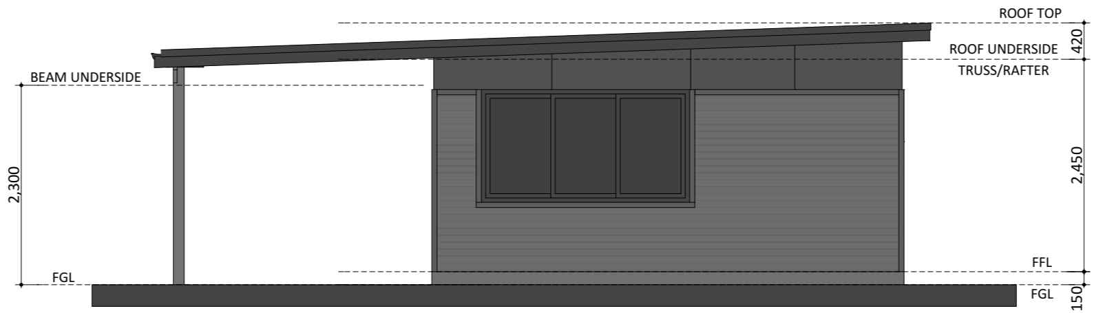
ELEVATION 02
