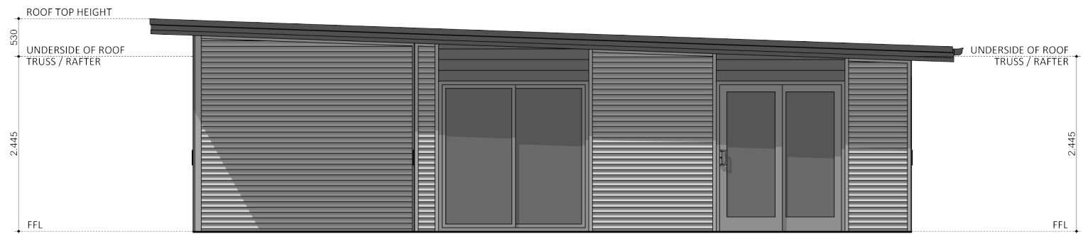
ELEVATION 02
