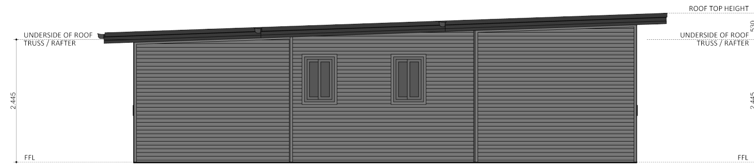
ELEVATION 04
