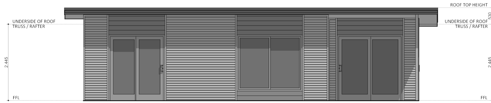
ELEVATION 01
