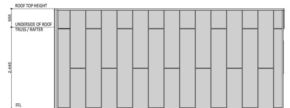
ELEVATION 04
