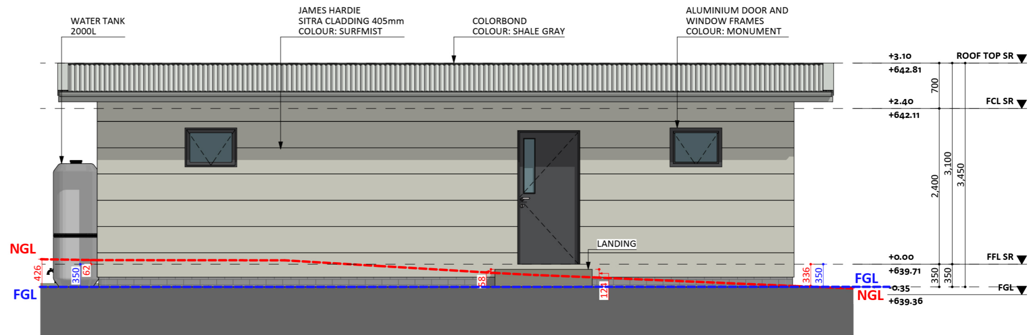
ELEVATION 04
