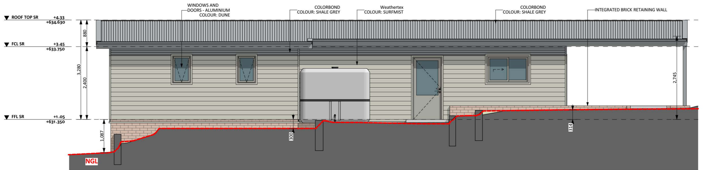
ELEVATION 04
