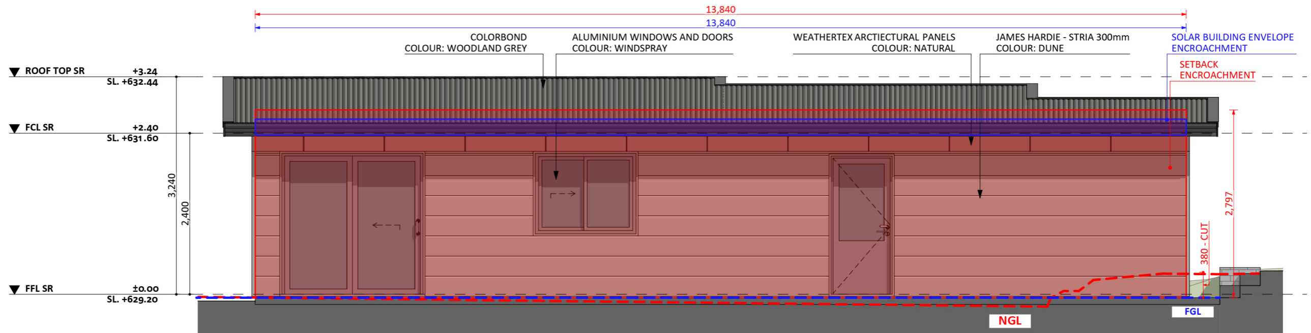
ELEVATION 04
