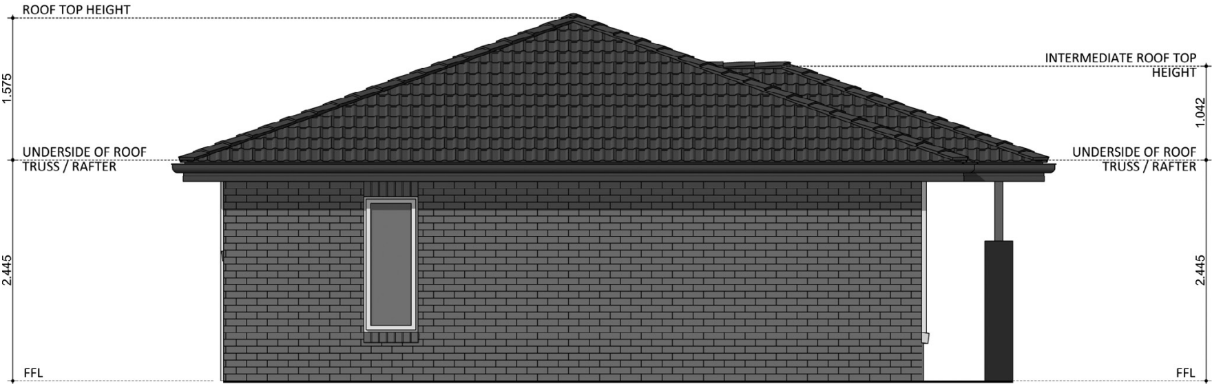
ELEVATION 02
