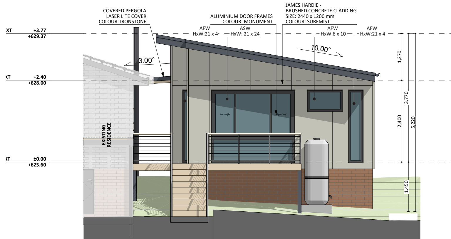
E3 WEST ELEV. - MR. 1:55
