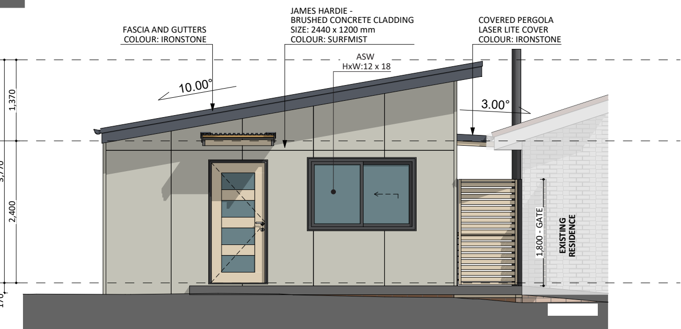
E4 EAST ELEV. - MR.
