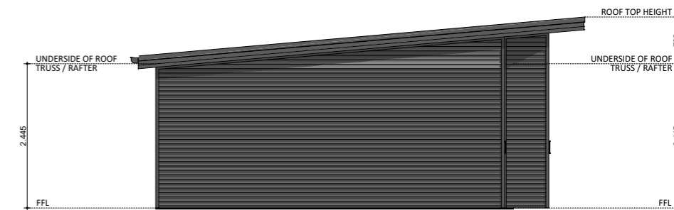
ELEVATION 04
