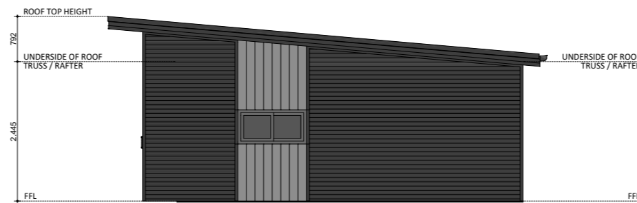
ELEVATION 02
