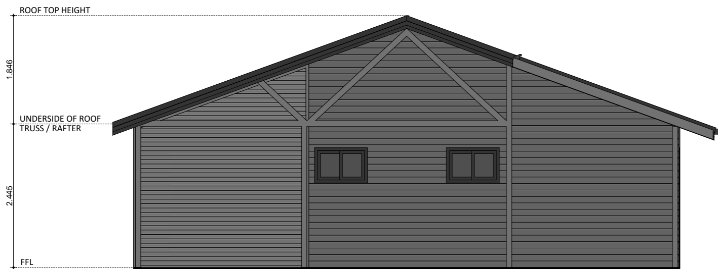
ELEVATION 02
