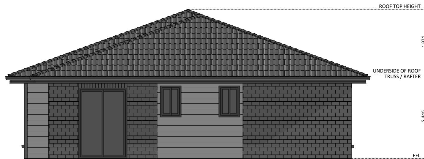
ELEVATION 04
