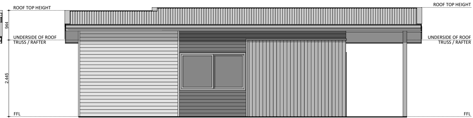
ELEVATION 04
