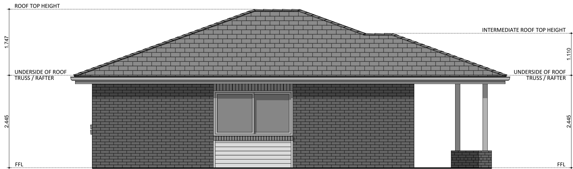
ELEVATION 04
