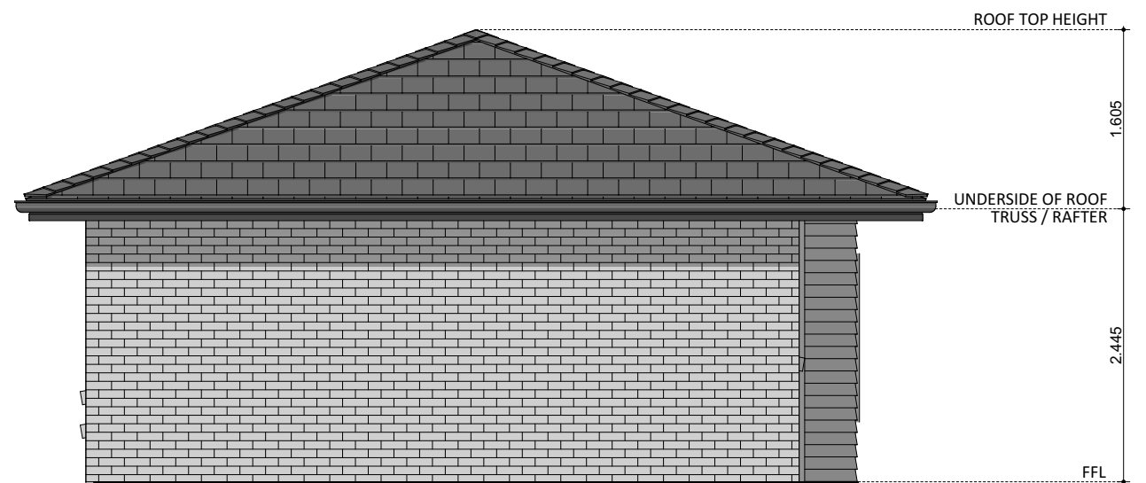
ELEVATION 04
