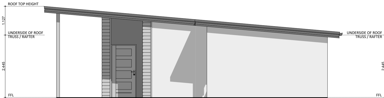
ELEVATION 02
