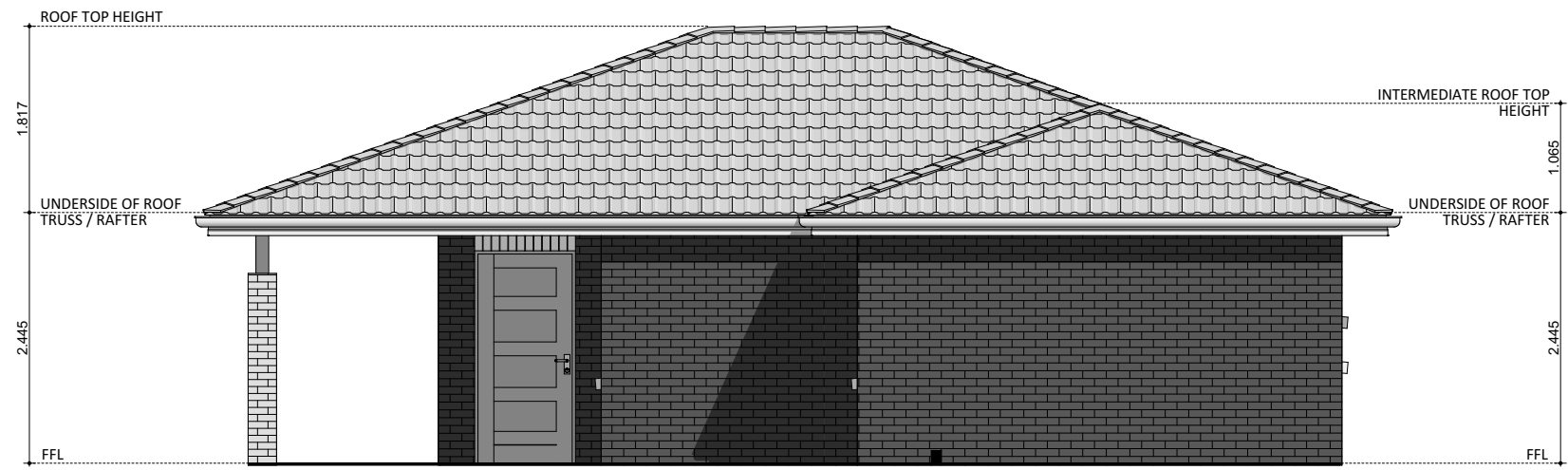
ELEVATION 02
