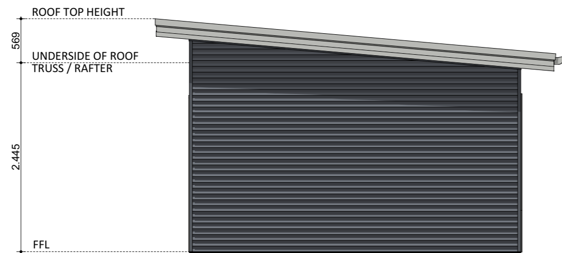
ELEVATION 02
