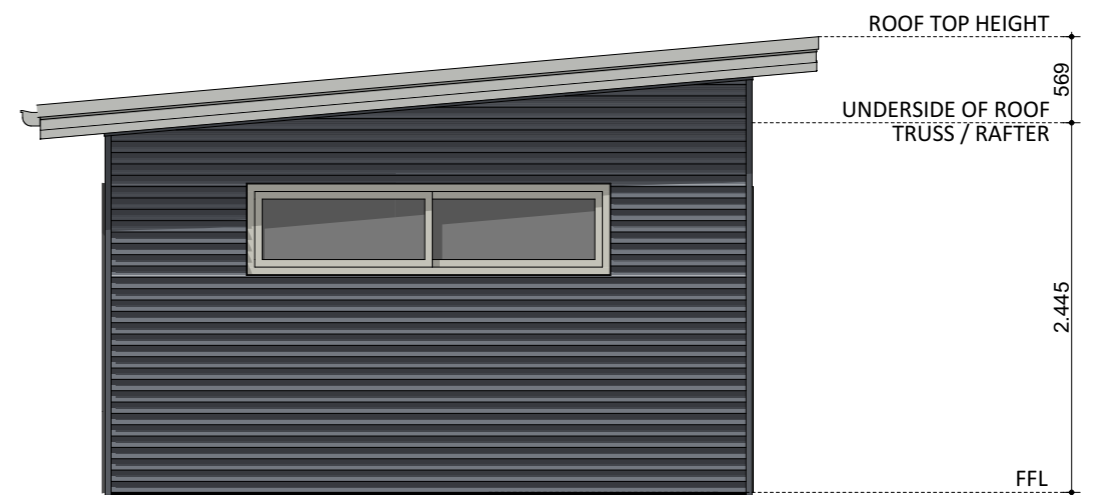
ELEVATION 04
