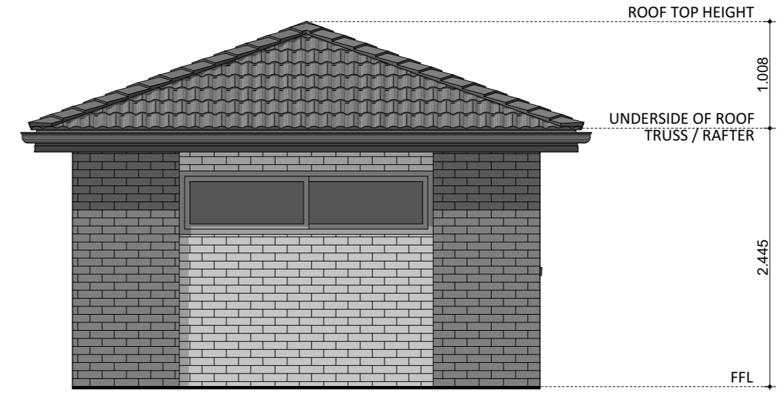
ELEVATION 04
