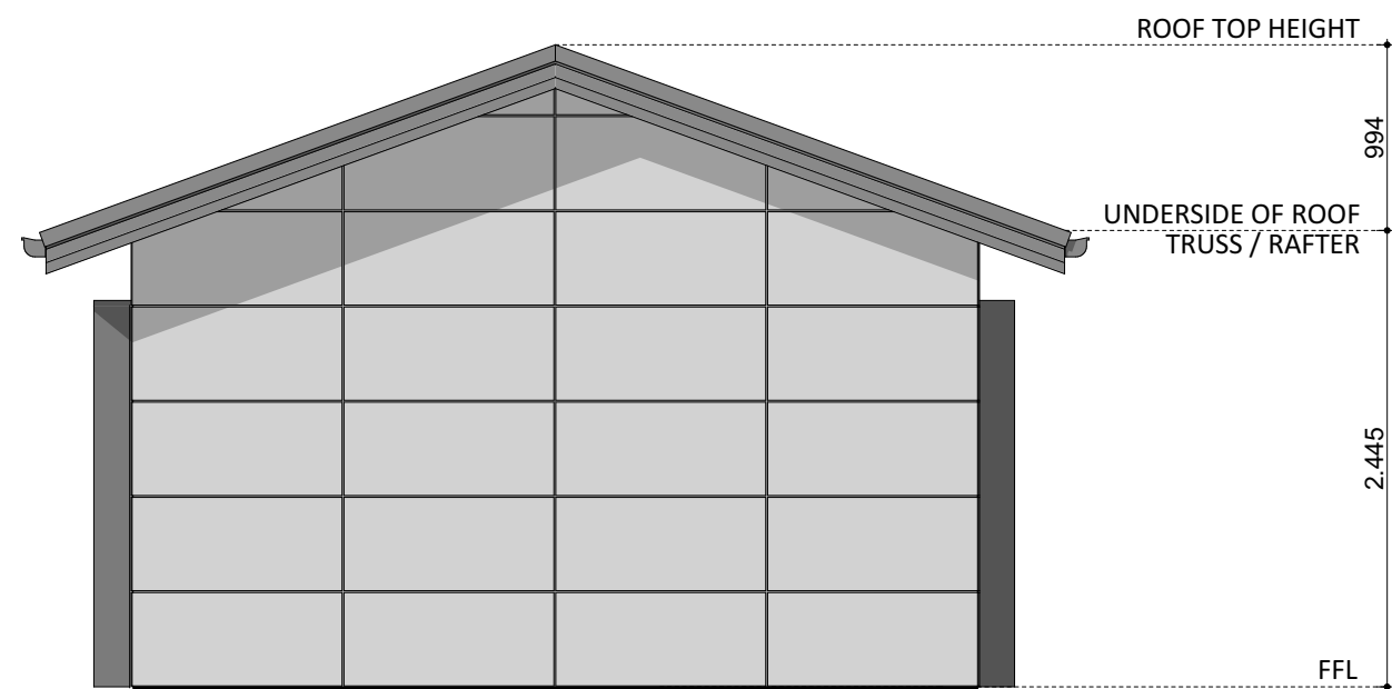
ELEVATION 04
