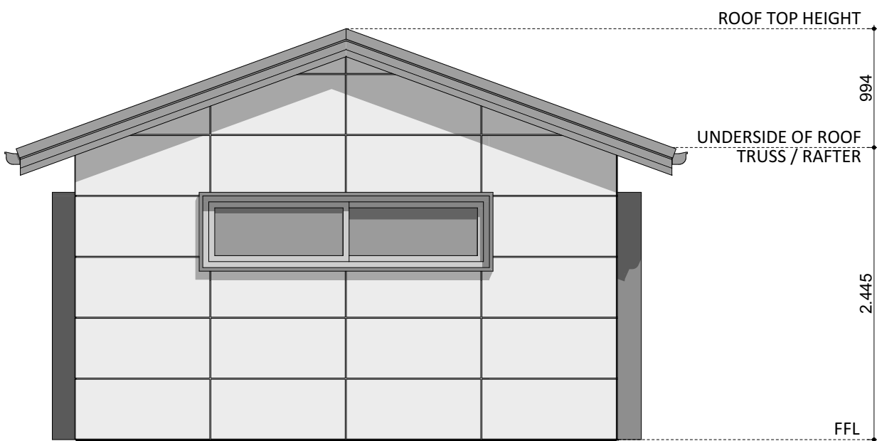
ELEVATION 02
