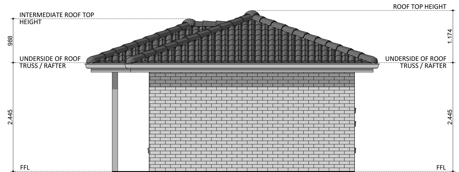
ELEVATION 04
