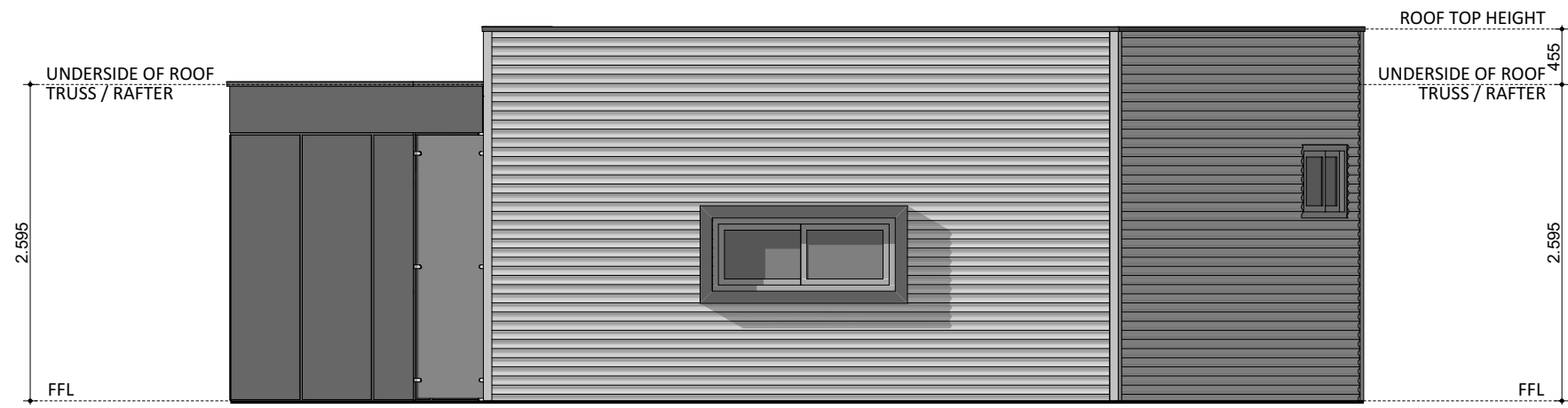
ELEVATION 01
