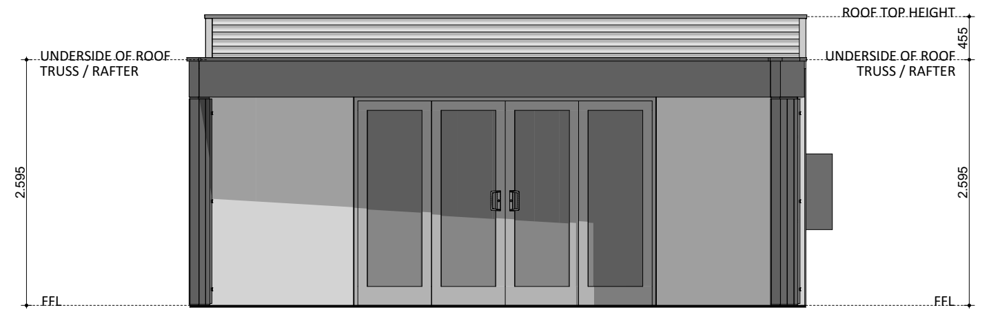
ELEVATION 04
