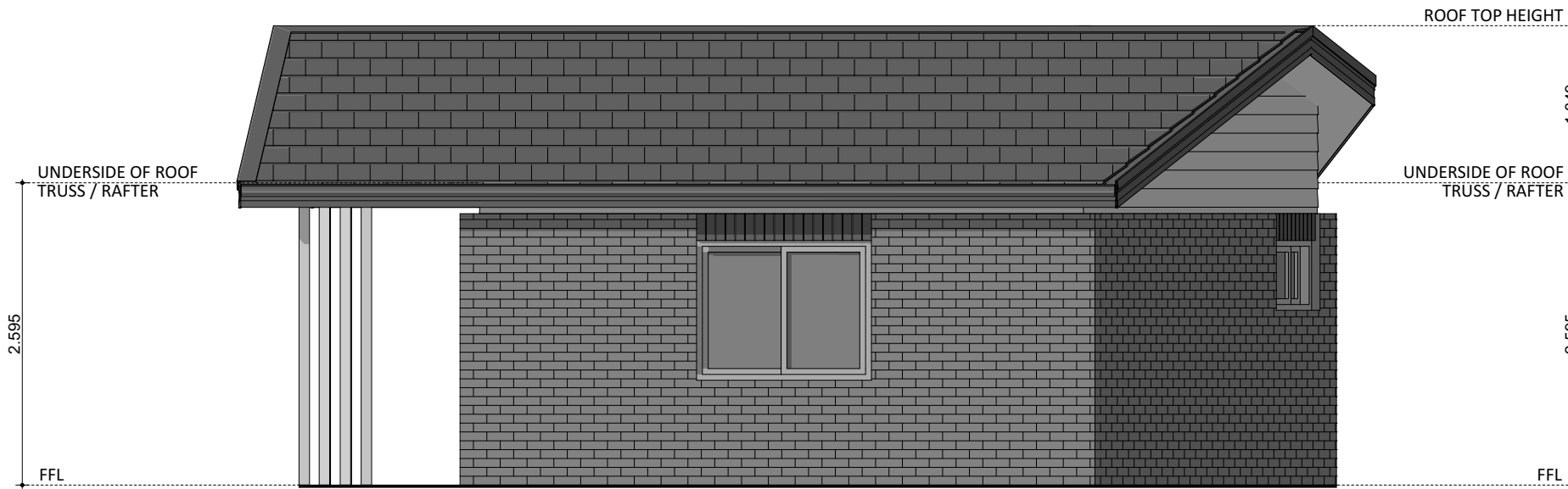
ELEVATION 01
