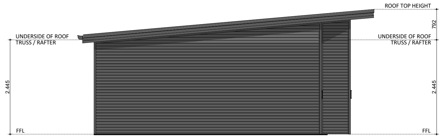
ELEVATION 04
