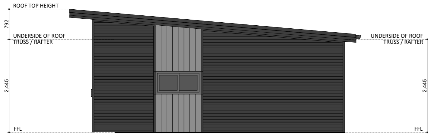
ELEVATION 02
