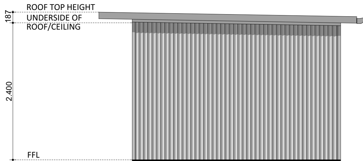
ELEVATION 02
