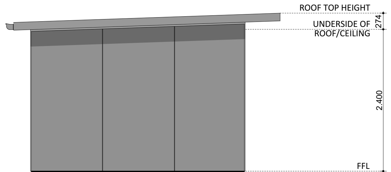
ELEVATION 04
