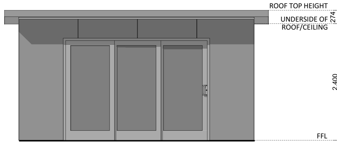
ELEVATION 01
