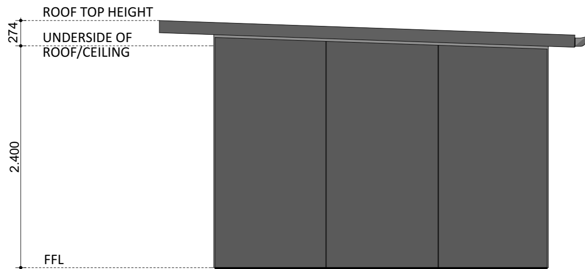
ELEVATION 02
