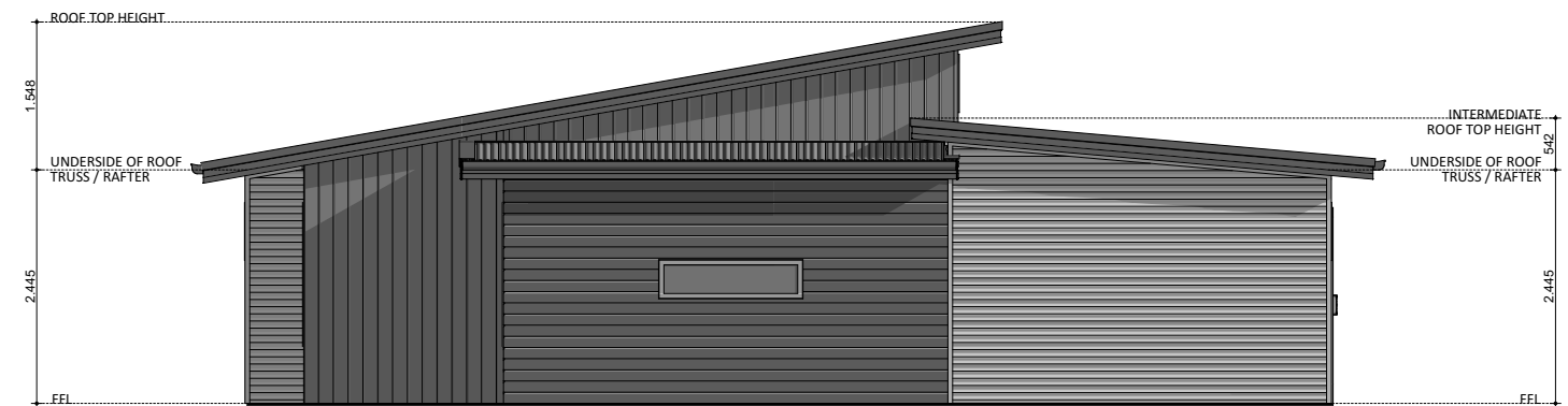
ELEVATION 04
