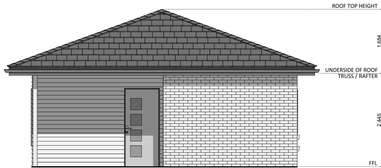
ELEVATION 02
