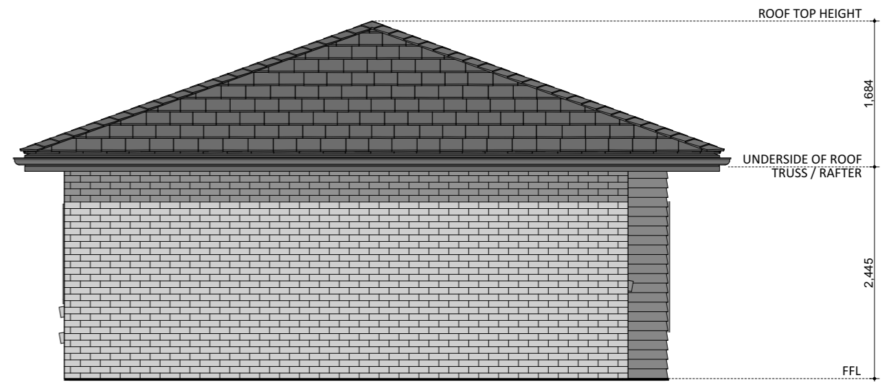
ELEVATION 04
