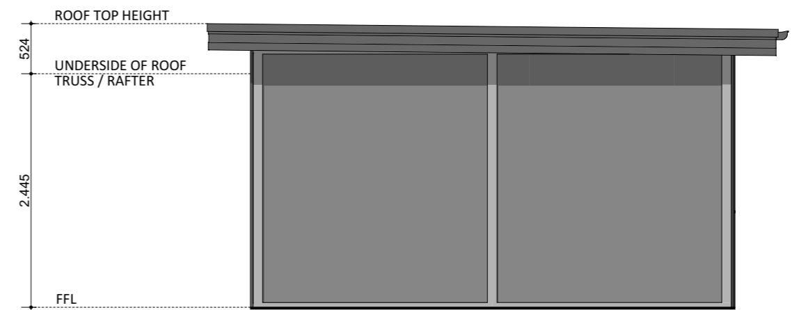
ELEVATION 04
