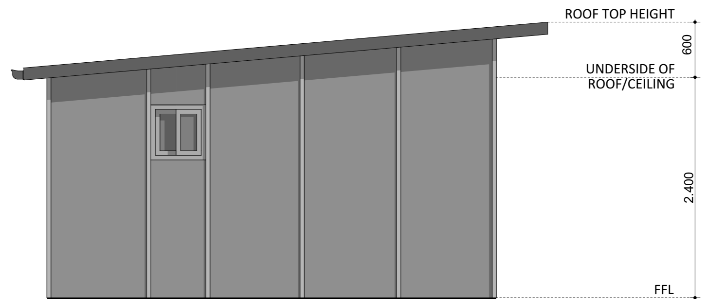
ELEVATION 04
