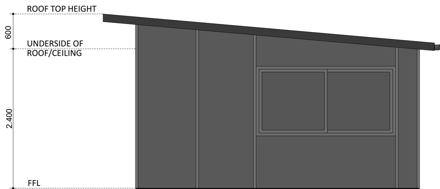
ELEVATION 02
