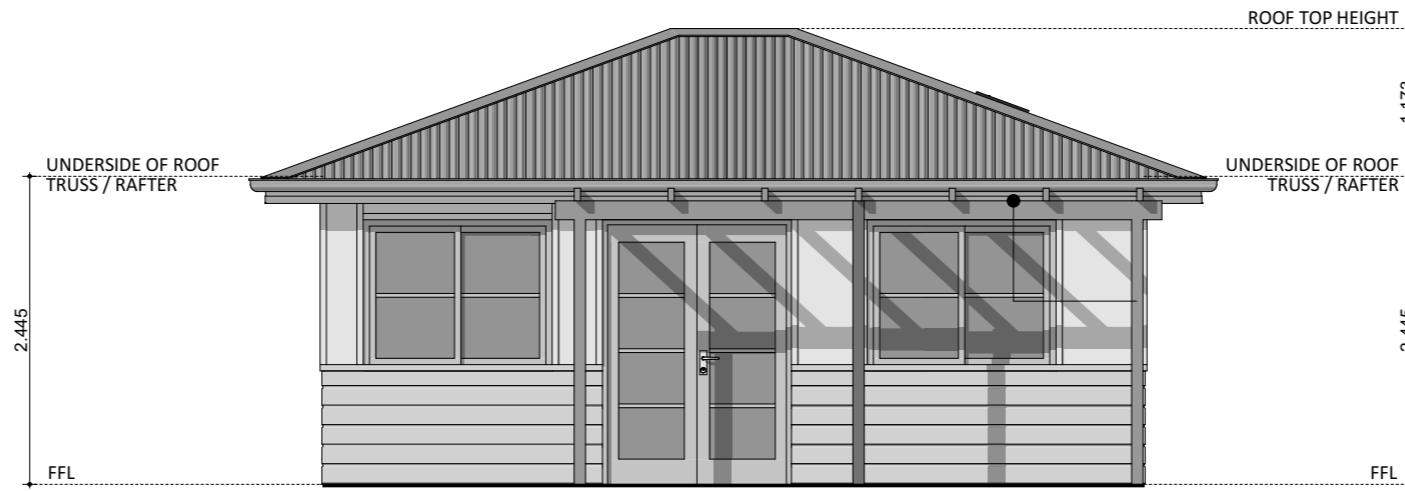
ELEVATION 01
