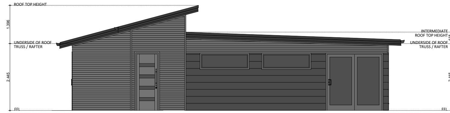
ELEVATION 04
