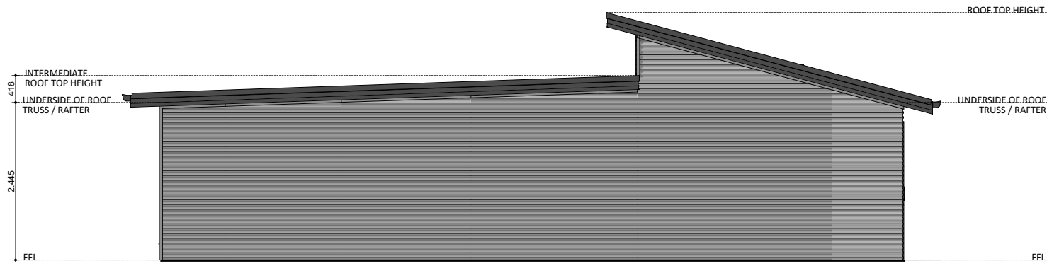
ELEVATION 02
