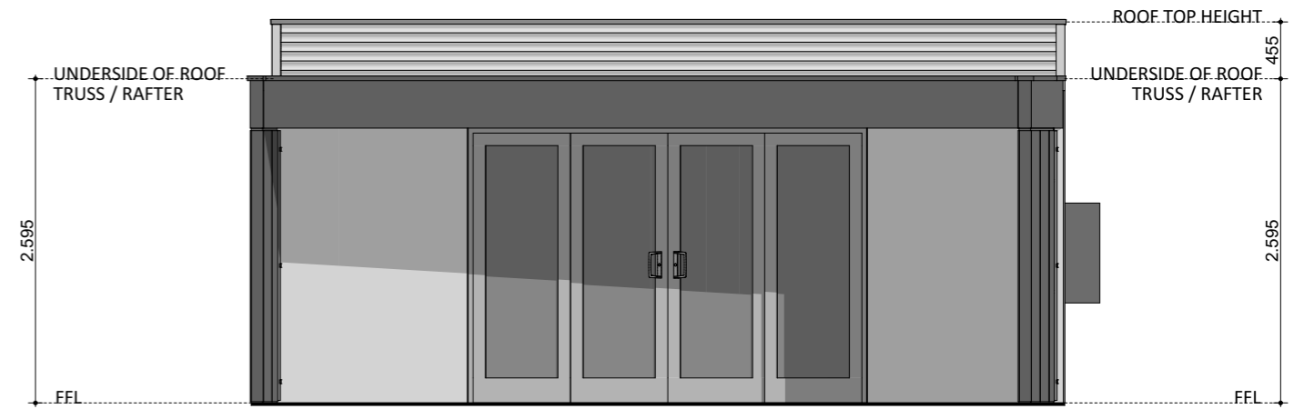
ELEVATION 04
