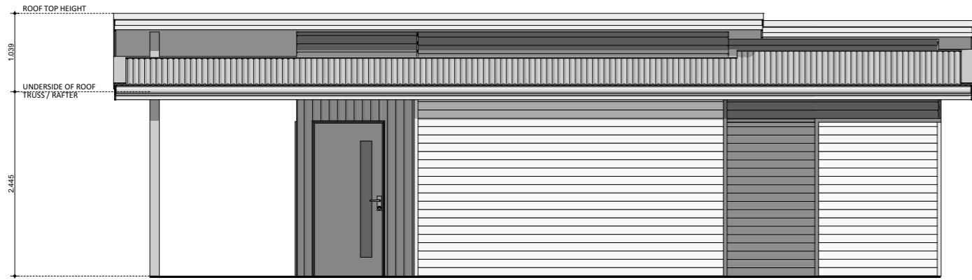
ELEVATION 02
