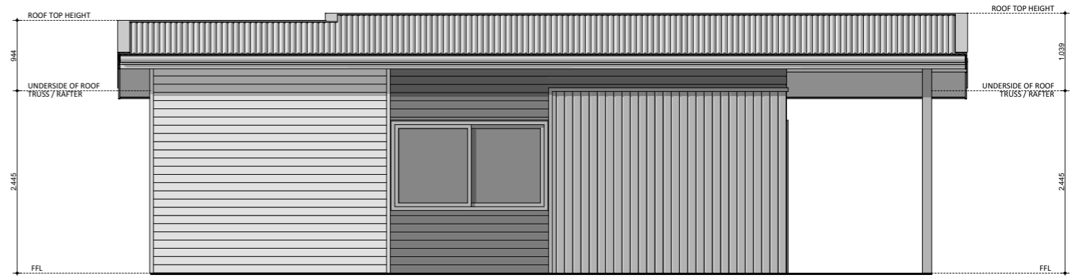
ELEVATION 04
