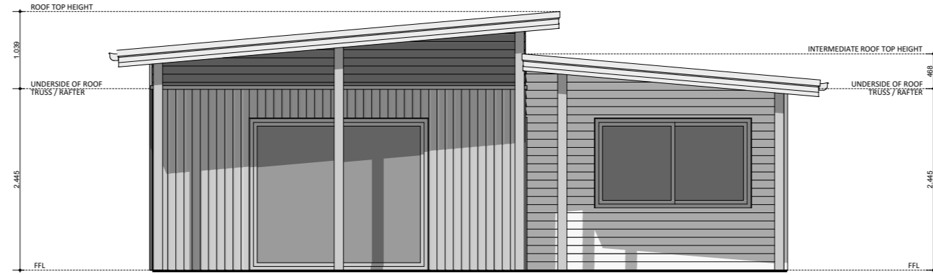
ELEVATION 01
