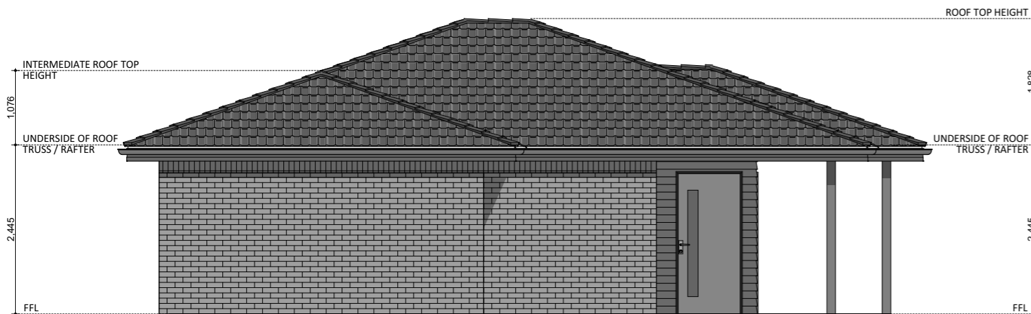
ELEVATION 02
