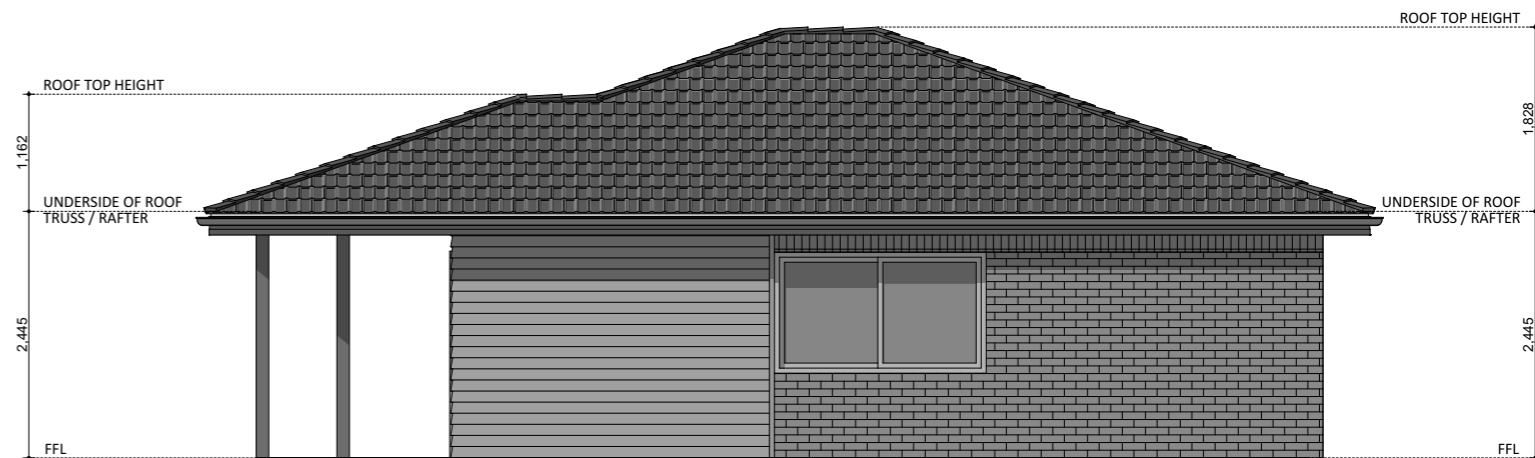
ELEVATION 04
