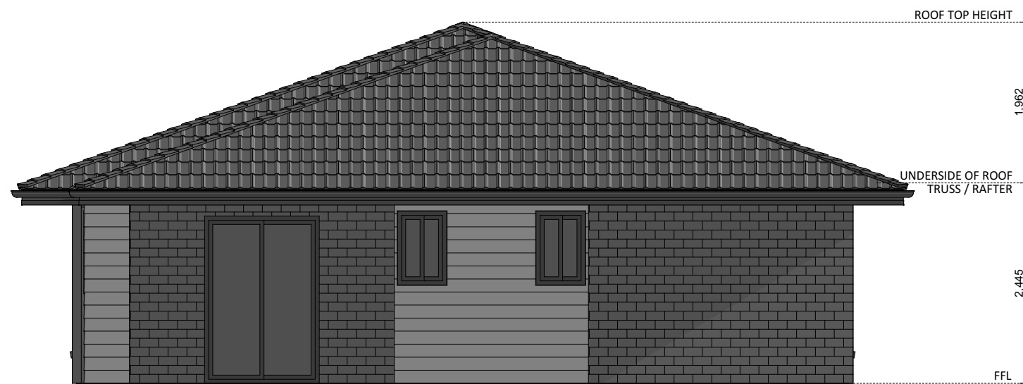
ELEVATION 04
