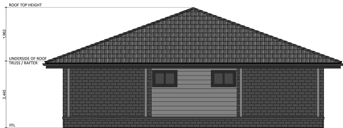
ELEVATION 02
