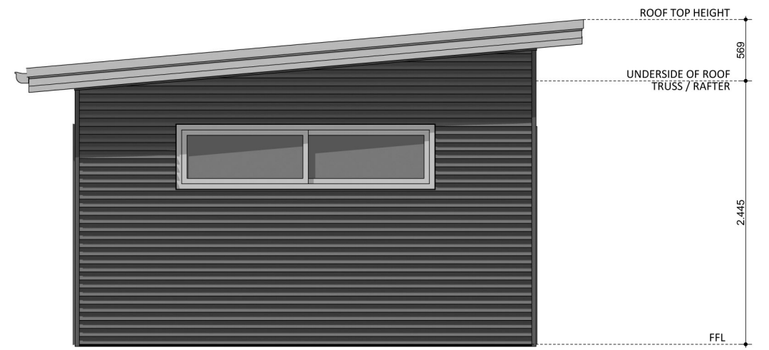
ELEVATION 04
