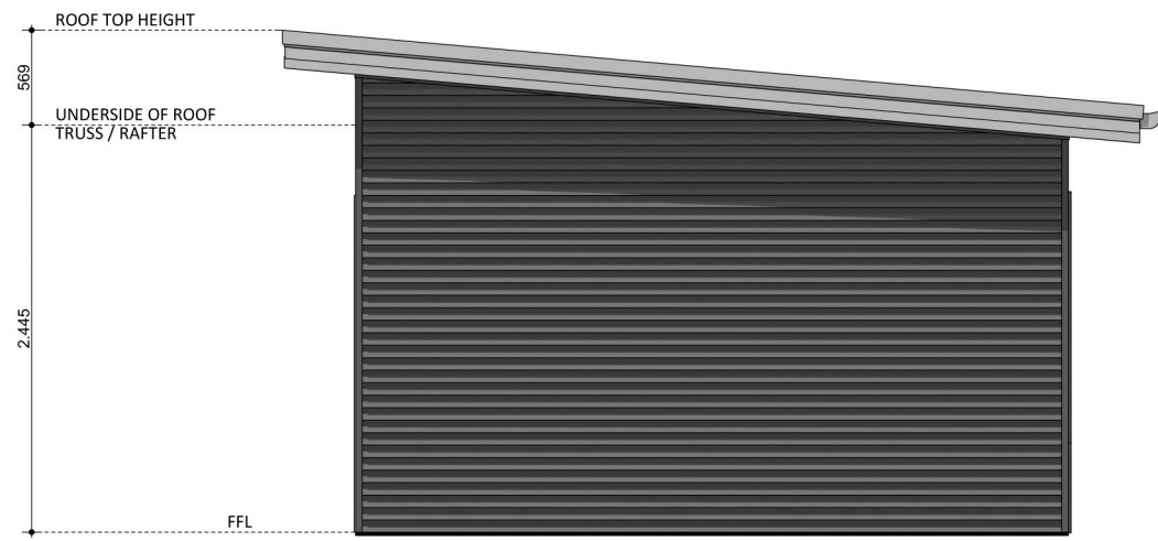
ELEVATION 02
