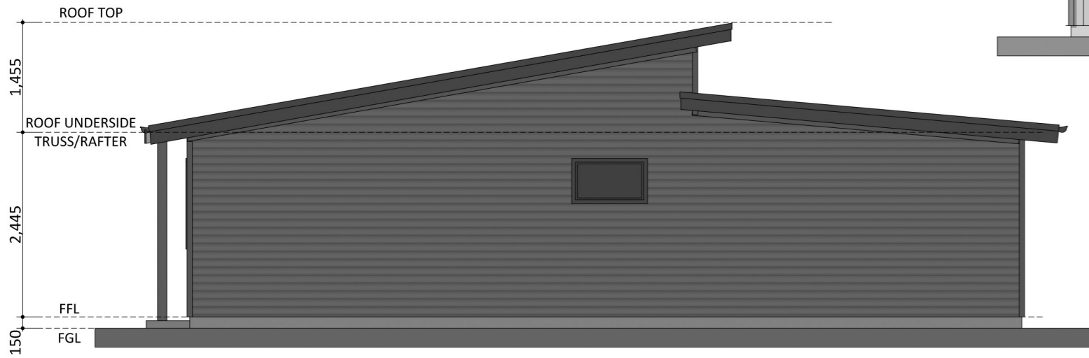
ELEVATION 3
