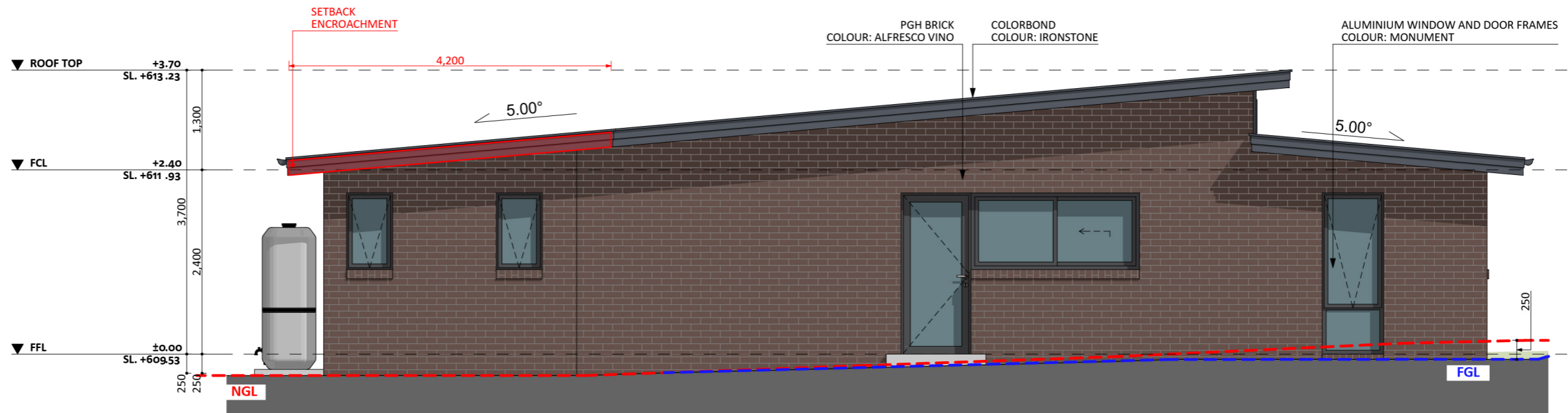
ELEVATION 04
